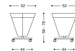
TRIANGLE CON RUOTE ● 3BR ● 3GR
